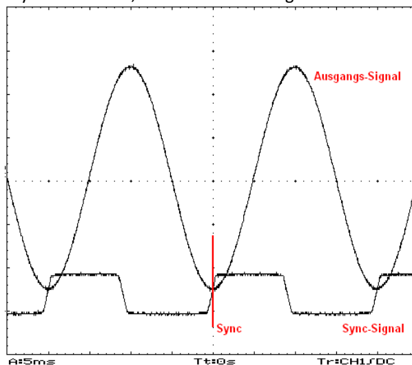
Synchronisation, Phasenverschiebung -90°
