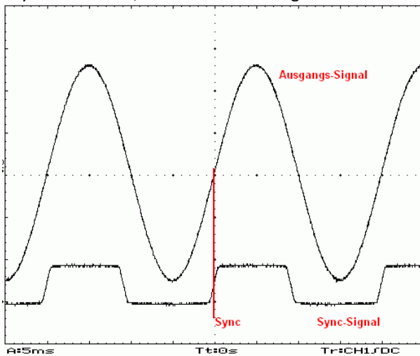
Synchronisation, Phasenverschiebung 0°
