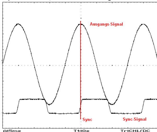
Synchronisation, Phasenverschiebung +90°
